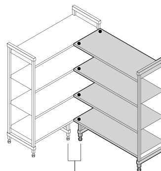
Под каждой базовой и дополнительной секцией используется одна напольная опора.
